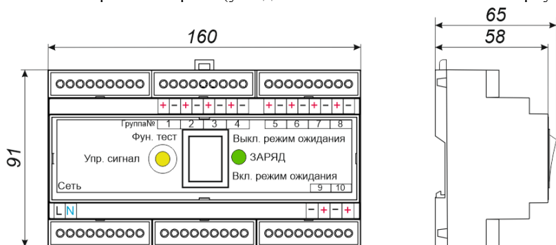
Рис. №1. Габаритный чертёж (у модели BS-TELECONTROL-2 на корпусе нет управляющей кнопки и индикаторов).
