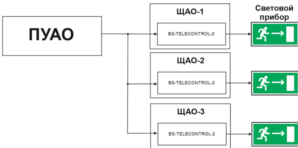
Рис №3. Схема подключения УДТУ BS-TELECONTROL-2 к ПУАО BS-ALARIS-1/3, для реализации Общего режима ожидания на объекте.
